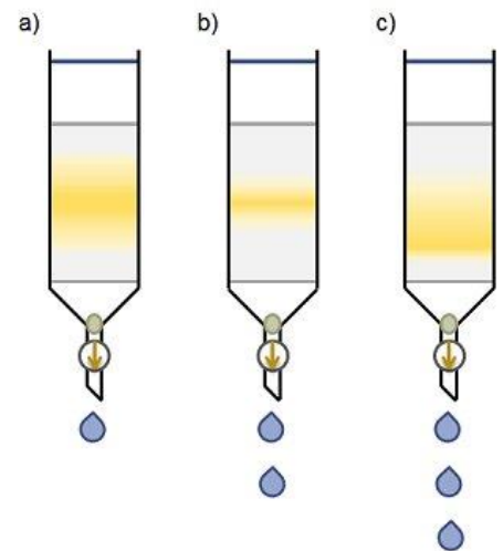
Figuur 3.31. De basis van een kolom. Door het type vloeistof wat gebruikt wordt en het materiaal in de kolom kun je bepalen welke stoffen blijven hangen en welke stoffen in je vloeistof terecht komen. Bron: http://www.chemistryviews.org/details/education/2345141/Tips_and_Tricks_for_the_Lab_Column_Troubleshooting_and_Alternatives.html
