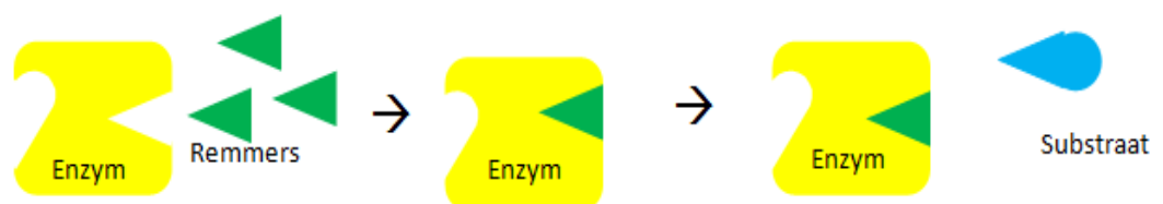
Figuur 3.39 Enzymremmer blokkeert de reactieplaats
